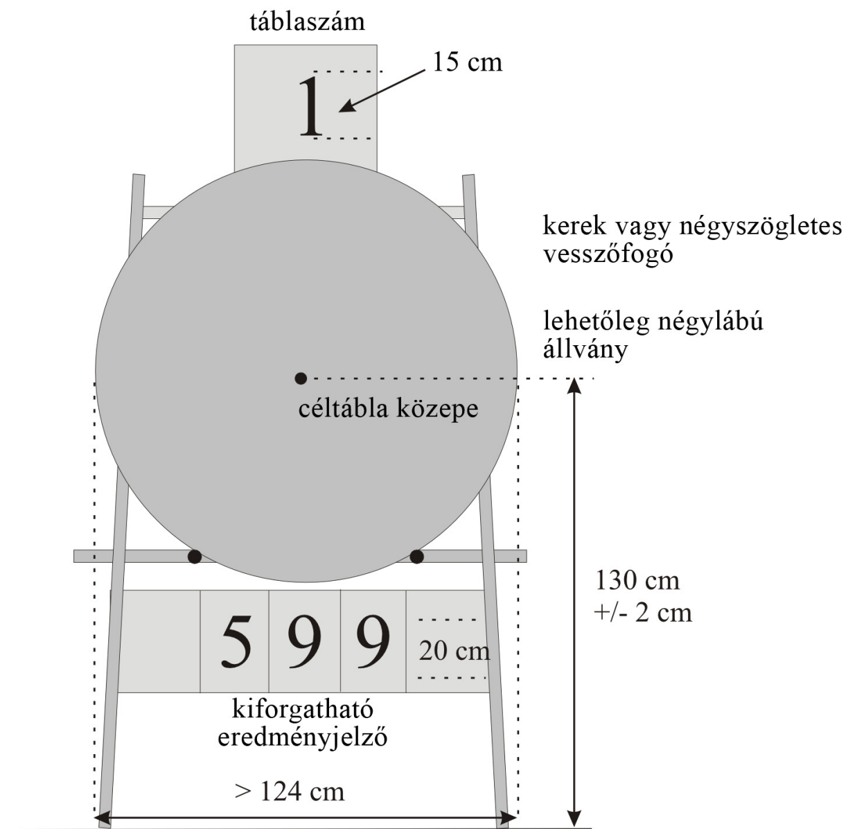
Image 10: Terem vesszőfogó
