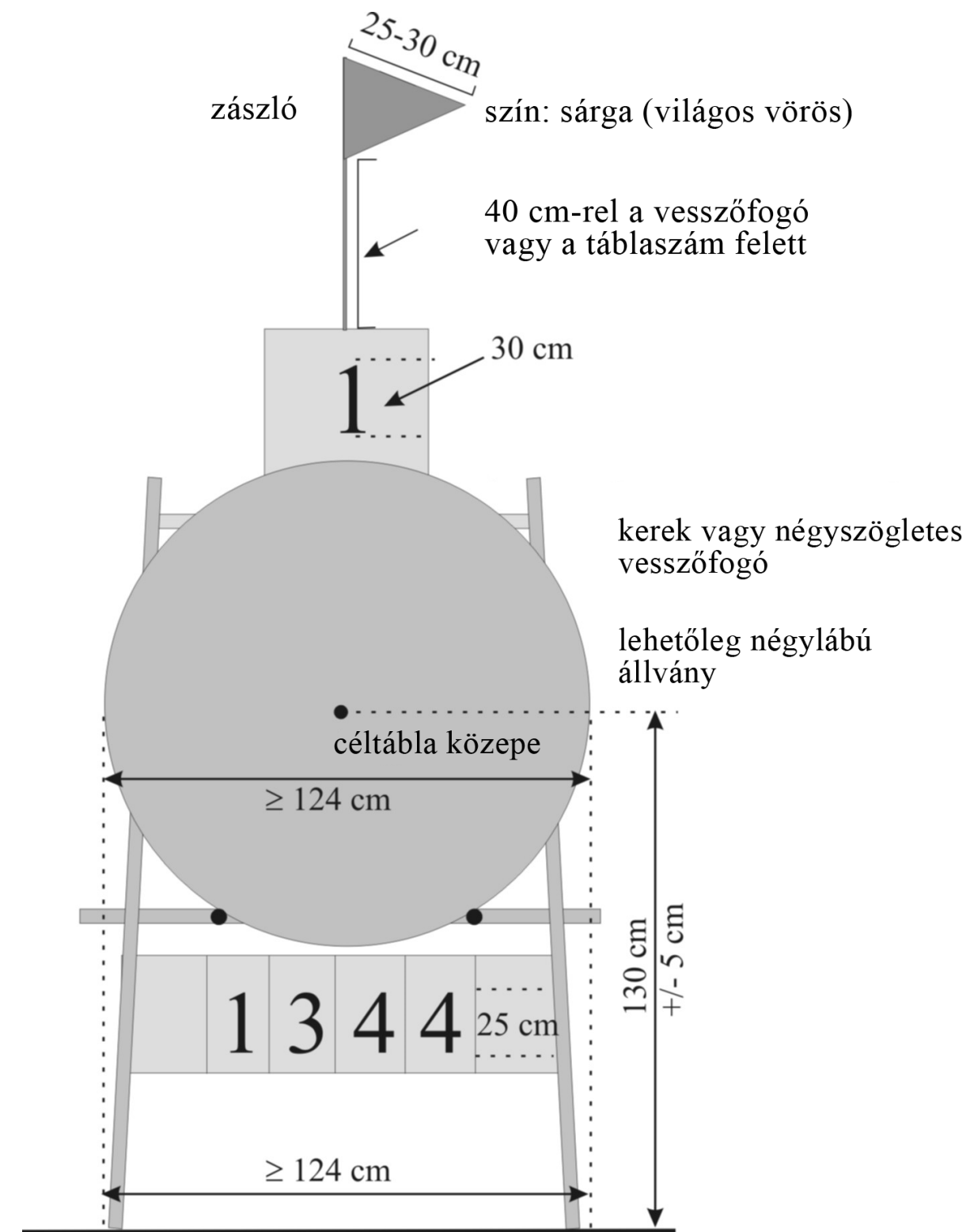
Image 3: Szabadtéri vesszőfogó
